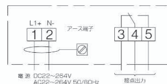
端子台部
